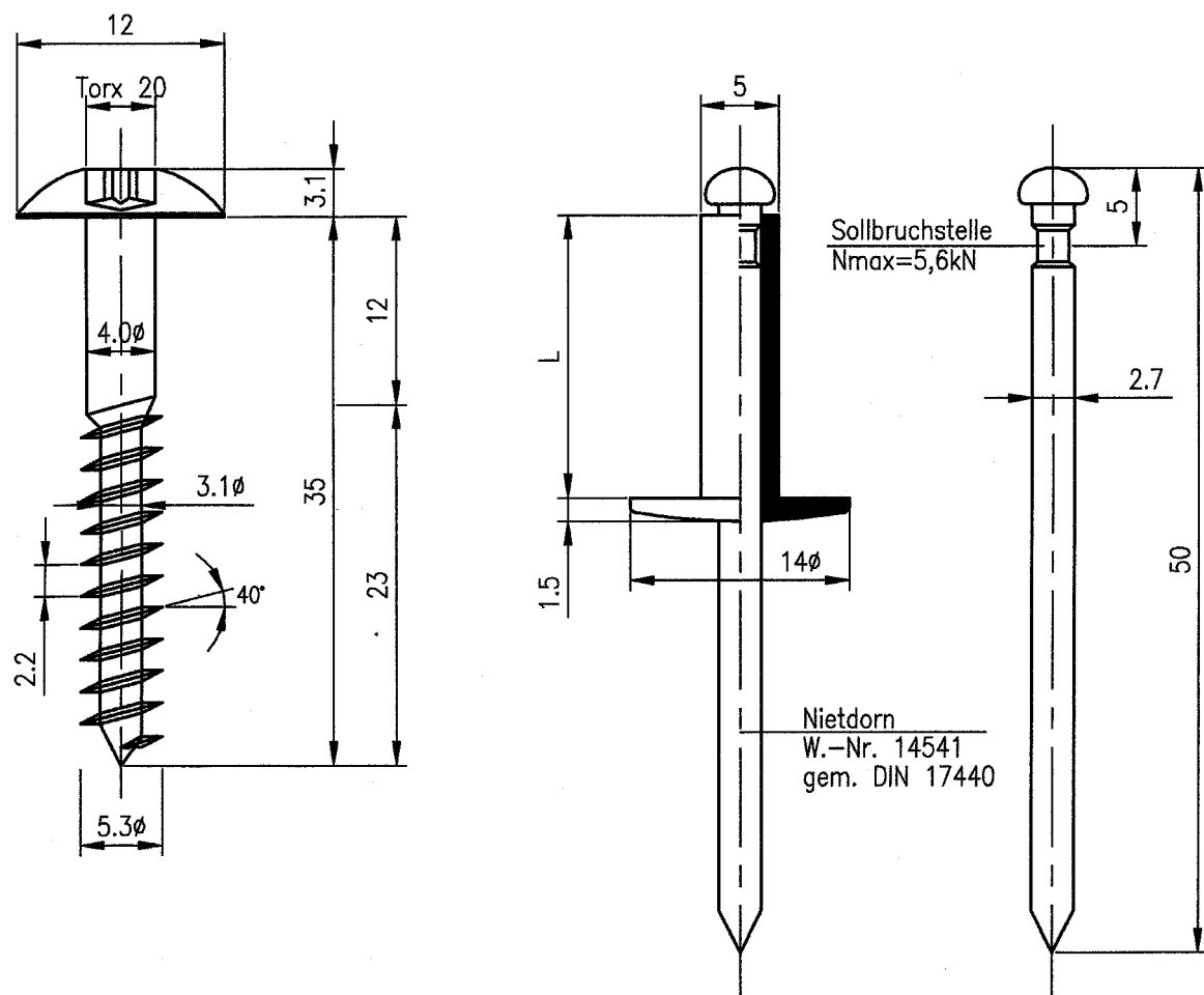
Fig. 2 : panneaux de façade MAX EXTERIOR - matériel de fixation
