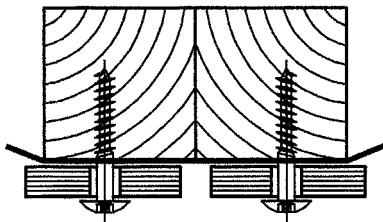
Coupe sur joint verticale bardage
