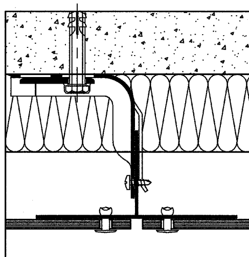
Fig. 3.4 : joint vertical (vue en coupe horizontale)
