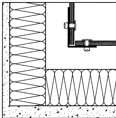
Fig. 3.6 : angle intérieur (vue en coupe horizontale)
