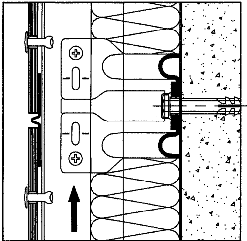
Fig. 3.1 : joint horizontal (vue en coupe verticale)
