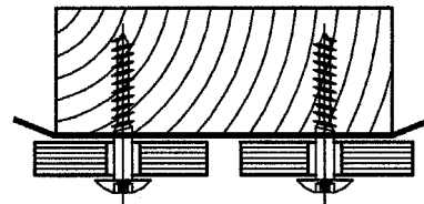
Doorsnede verticale voeg bekleding
