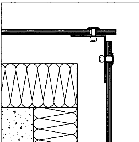
Fig. 3.5 : buitenhoek (horizontale doorsnede)
