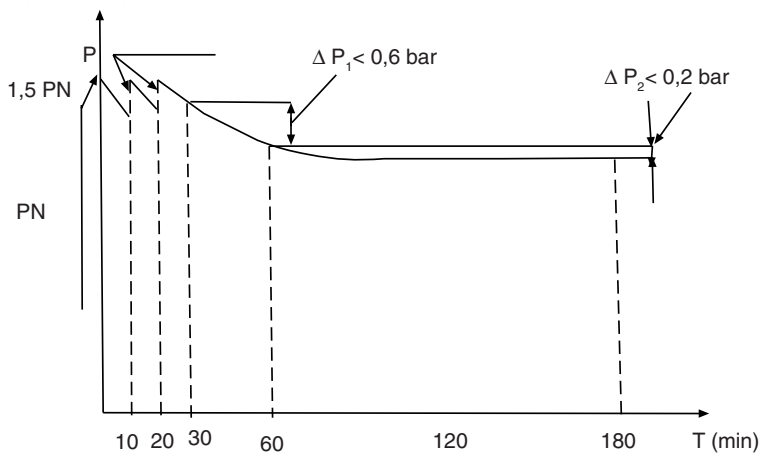
Fig. 6 : Diagramma dichtheidsbeproeving
