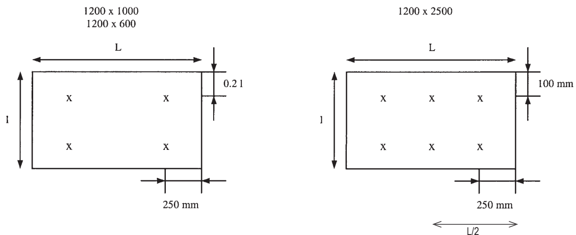
Fig. 2 : Plaatsing bevestigers voor mechanisch bevestigde platen
