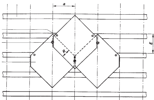
Fig. 4 : Ruitdekking
