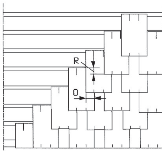
Fig. 2 : Dubbele dekking met open voeg R : verticale overlapping O : zijdelingse overlapping
