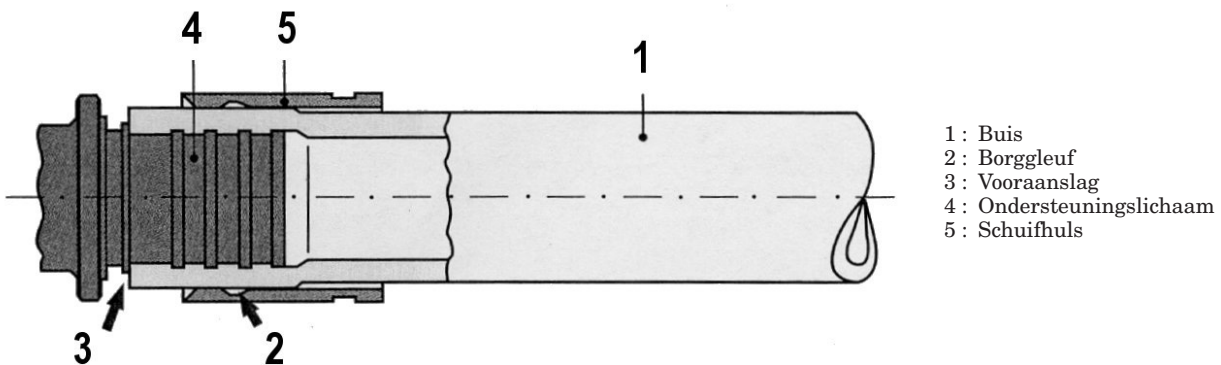
Fig. 1 : Schematische voorstelling koppelstuk met schuifhuls
