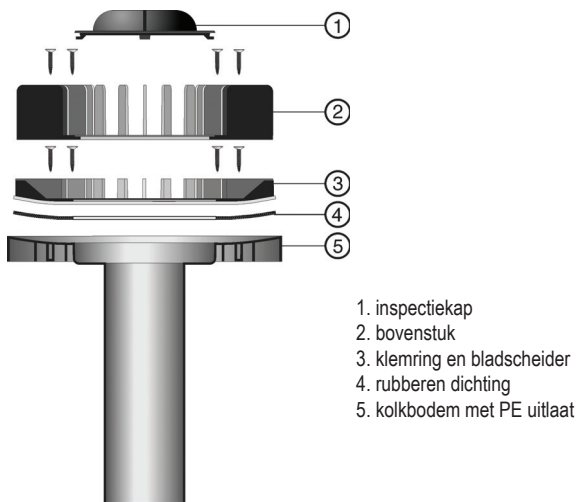
Fig. 1 : dakkolk voor klemmontage
