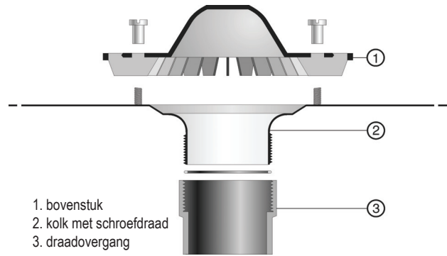
Fig. 3 : dakkolk voor bitumenmontage
