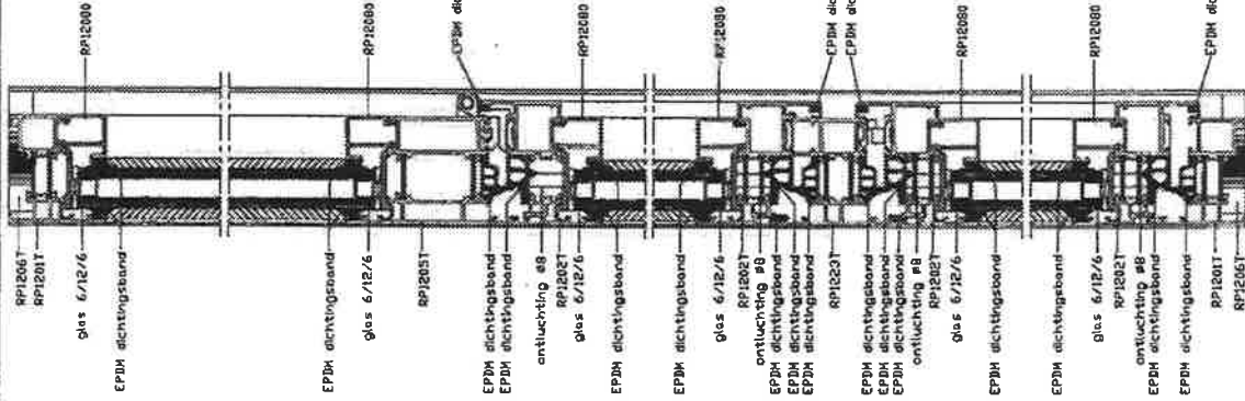
DOORSNEDE B-B
