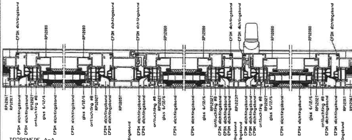
DOORSNEDE A-A
