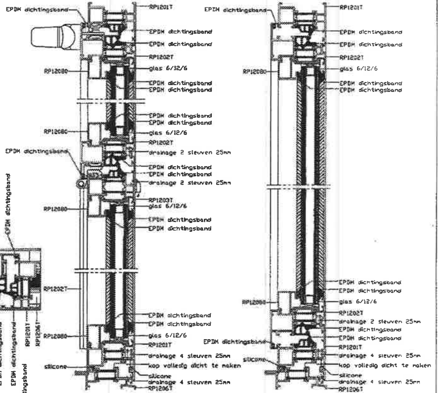
DOORSNEDE C-C
