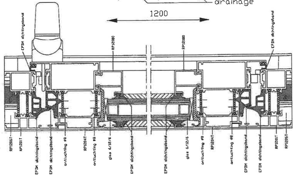
DOORSNEDE A-A
