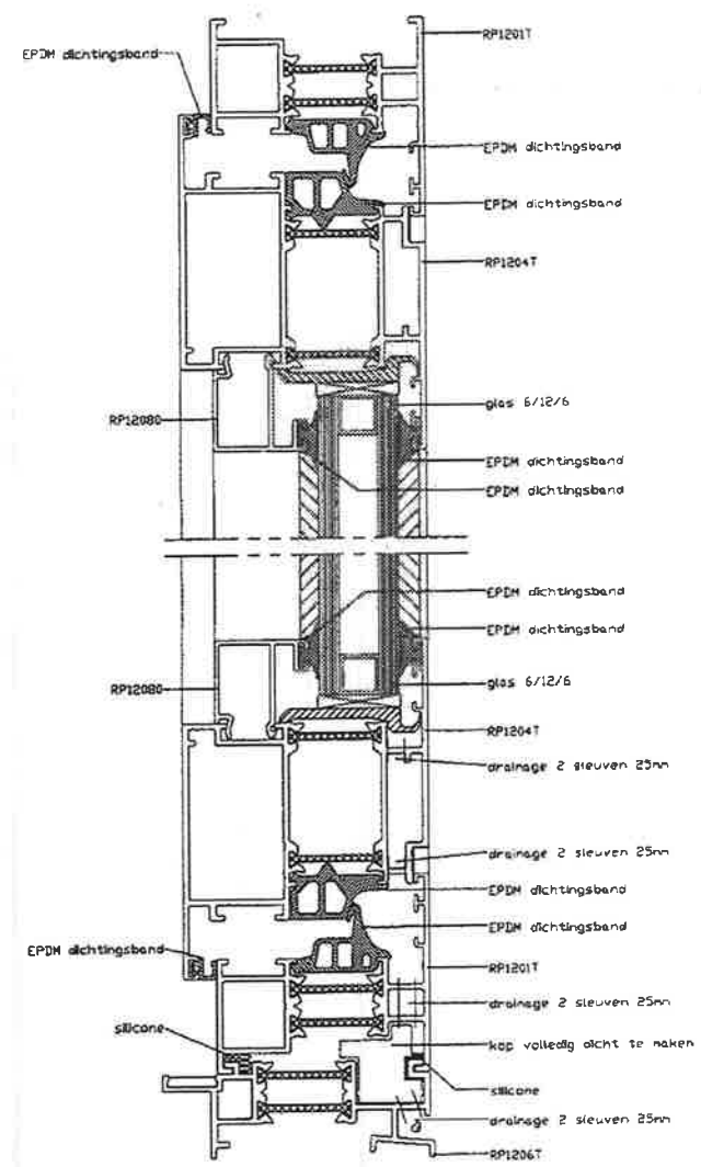
DOORSNEDE B-B
