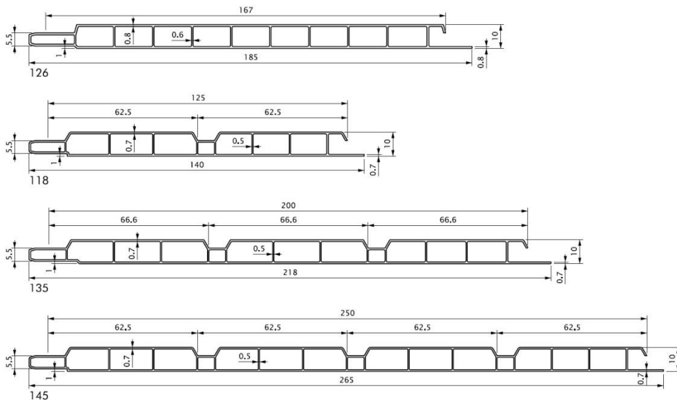
Figuur 2 – Gootbekledingsprofielen
