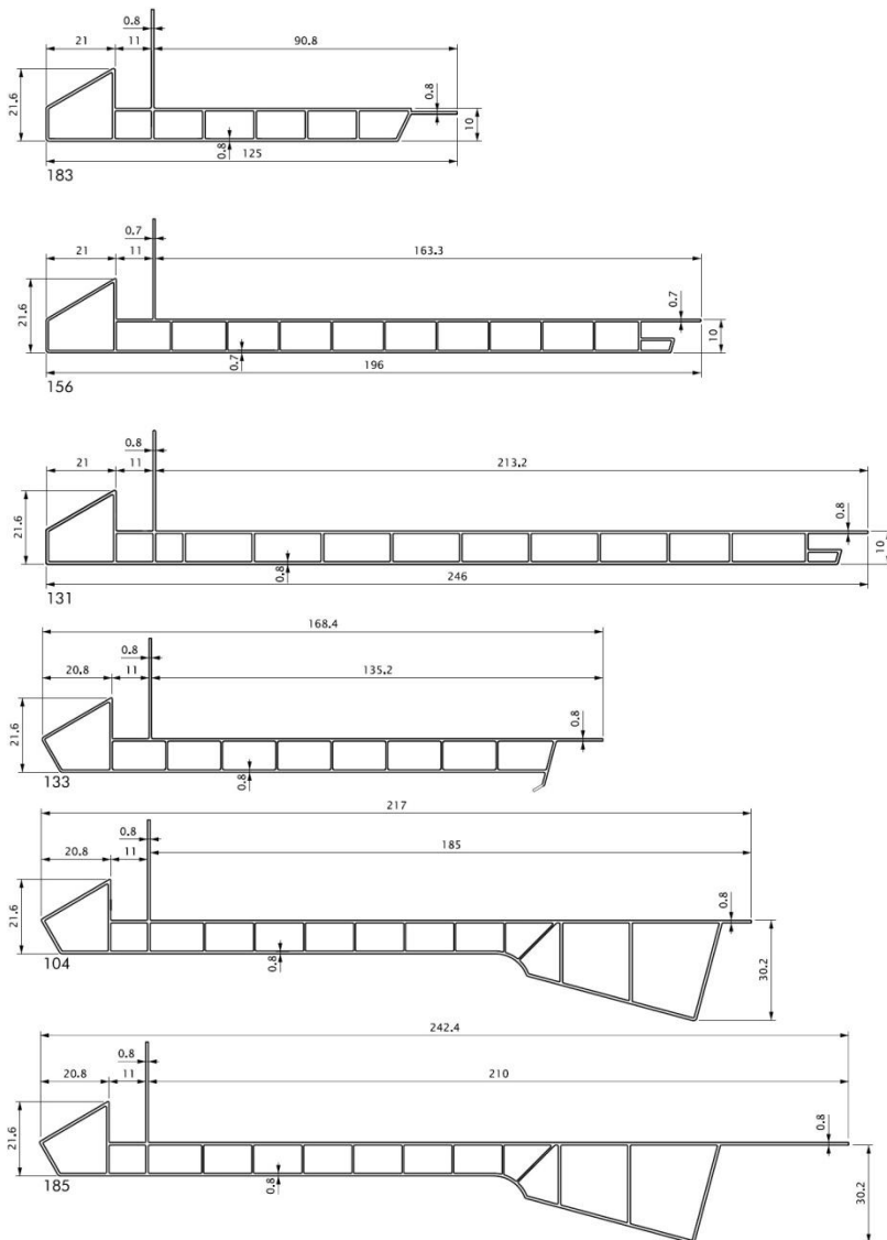
Figuur 2 – Gootbekledingsprofielen
