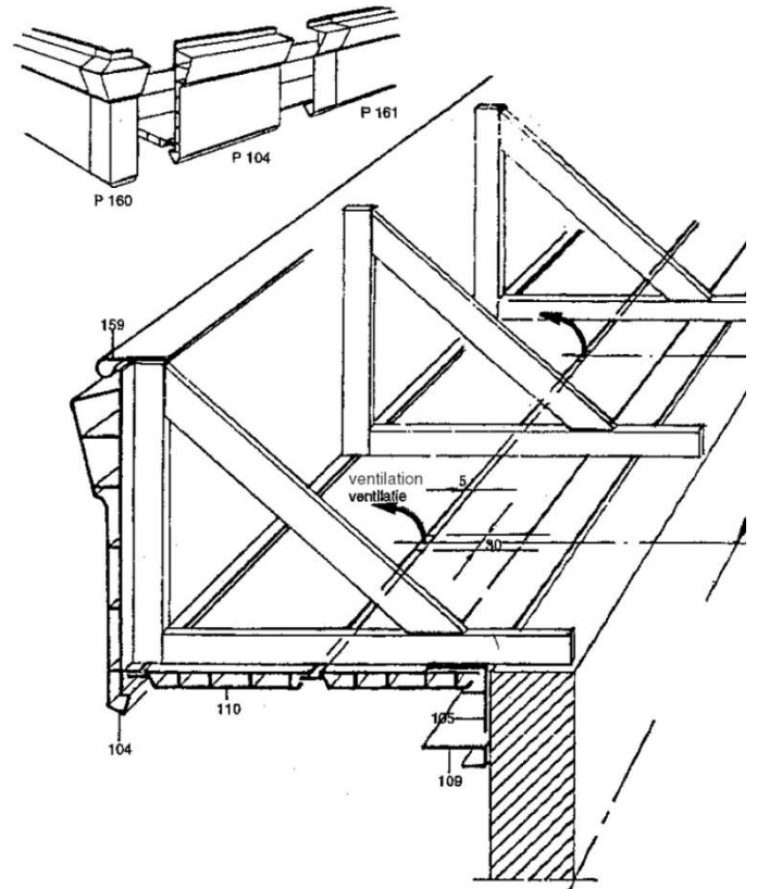
Figuur 6 – Plaatsingsvoorschriften gootbekledingsprofielen
