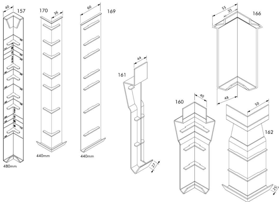
Figuur 4 – Spuitstukken
