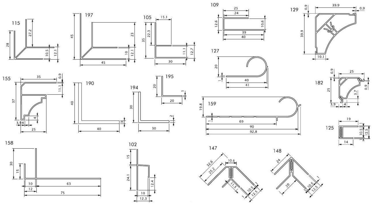
Figuur 3 (vervolg) – Afwerkingsprofielen
