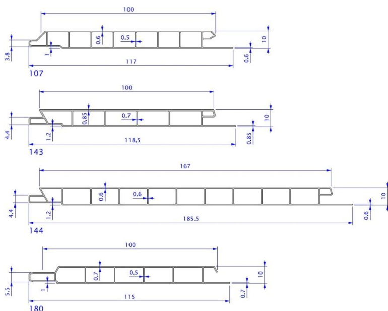
Figuur 1 – Bekledingsprofielen
