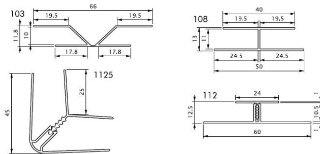
Figuur 4 – Spuitstukken
