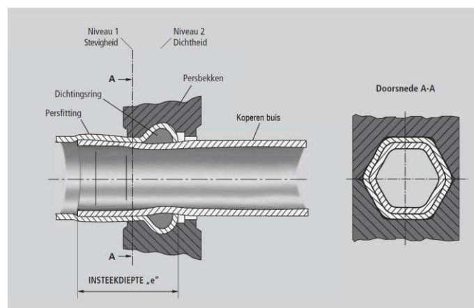
Fig. 1: lange doorsnede vóór en na het persen
