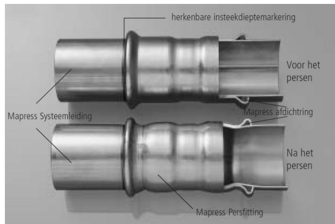
Fig. 1: lange doorsnede vóór en na het persen
