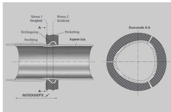
Fig. 3: dwarse doorsnede tijdens het persen (persketting)
