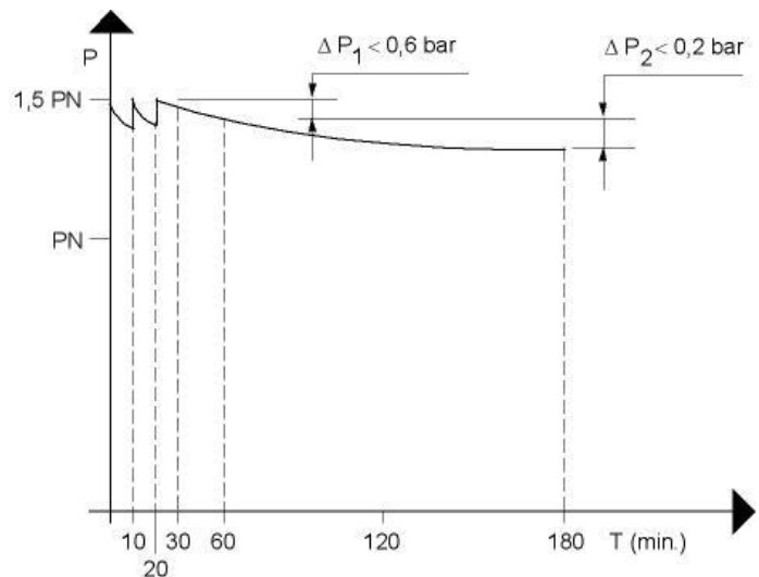
Fig. 5: procedure voor de dichtheidscontrole
