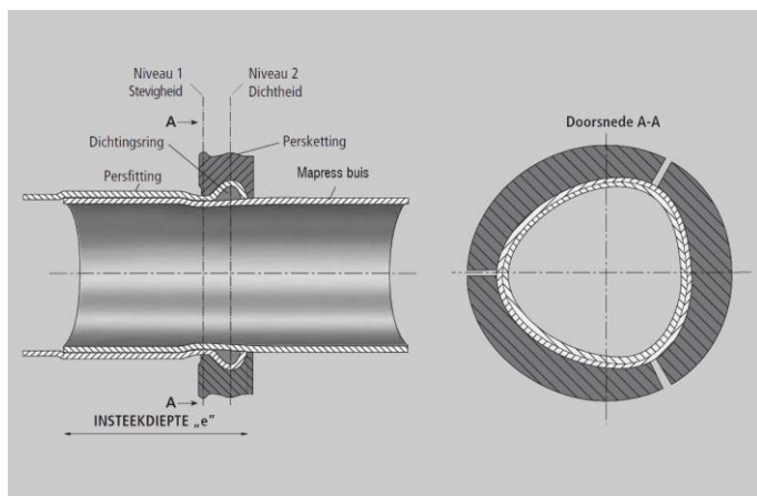
Fig. 3: dwarsdoorsnede tijdens het persen (persketting)
