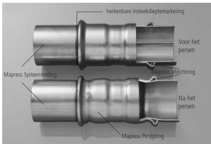
Fig. 1: langse doorsnede vóór en na het persen
