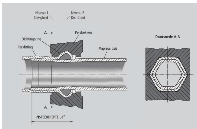
Fig. 2: dwarse doorsnede tijdens het persen (persklem)
