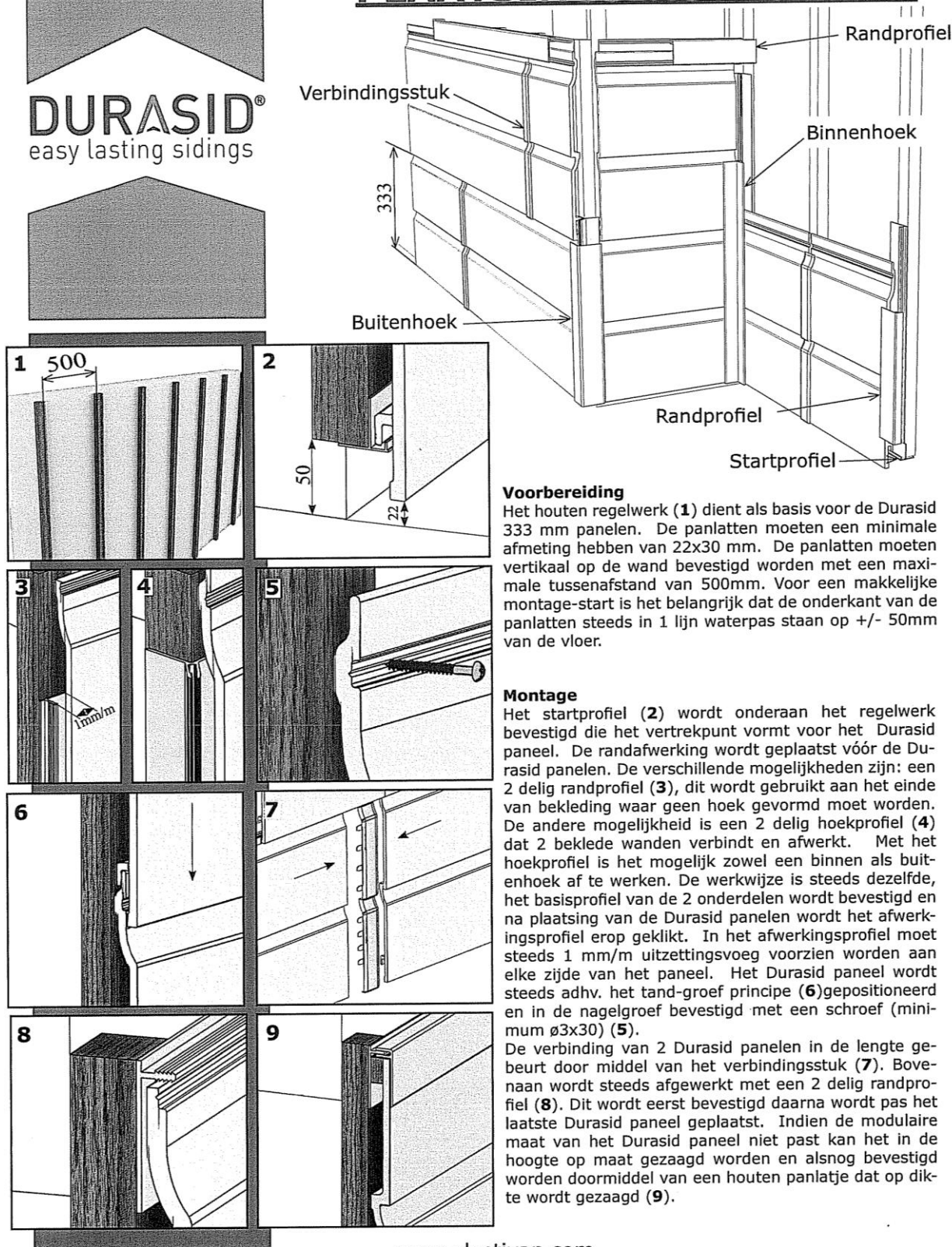
Fig. 6: Verschillende randafwerkingen voor het profiel 333
