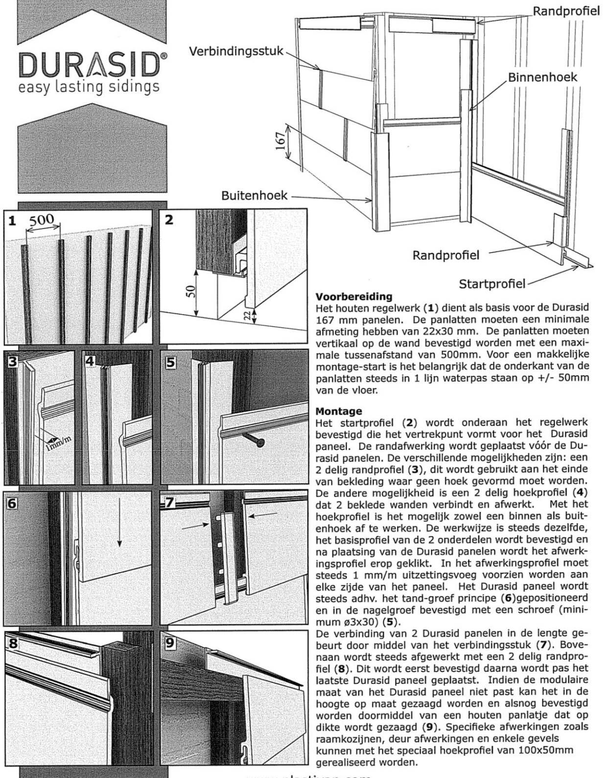
Fig. 7: Verschillende randafwerkingen voor het profiel 167
