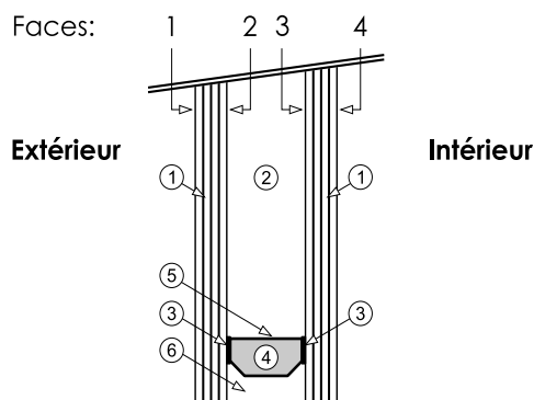
Figure 1 – Faces dans un vitrage isolant
