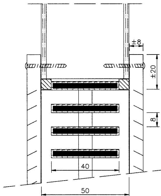
Snede C-C
