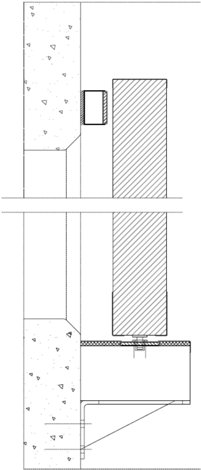
Figuur 8b : Haakslot Horizontale doorsnede
