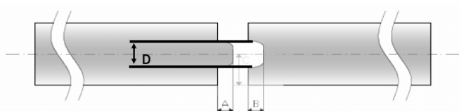
Figuur 1 – Tand- en groefverbinding
