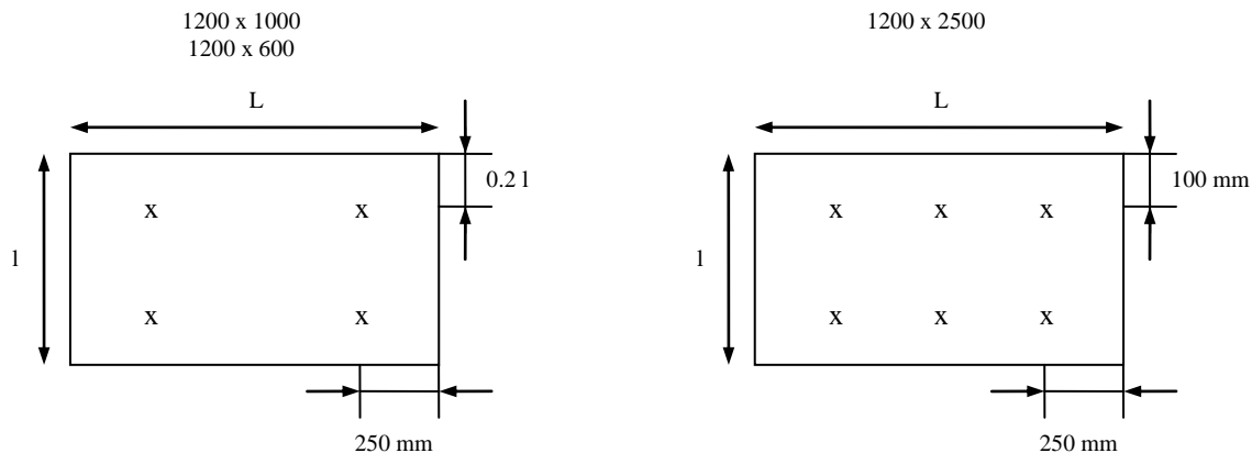
Fig. 2: Plaatsing bevestigers voor mechanisch bevestigde platen
