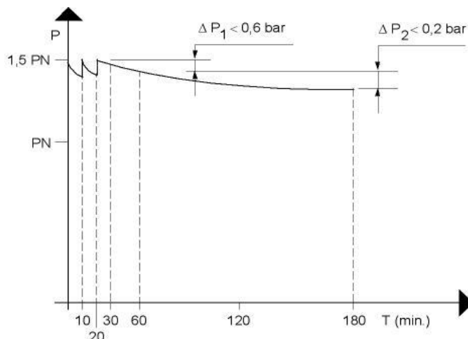
Fig. 1: — Contrôle d'étanchéité
