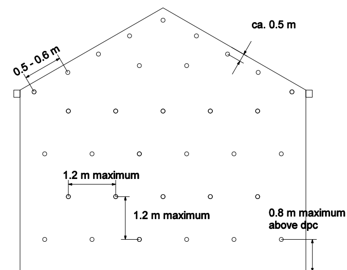
Figuur 1: Schematische weergave van het vulpatroon
