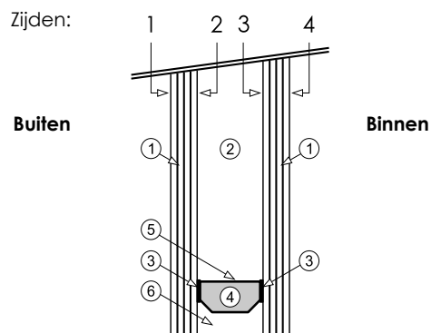
Figuur 1 – Kanten van een isolerende beglazing
