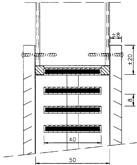
Coupe C-C
