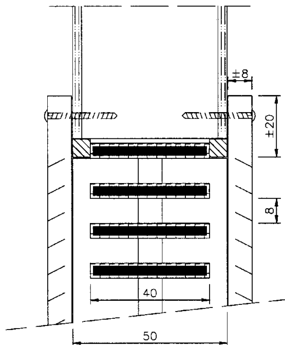
Snede C-C
