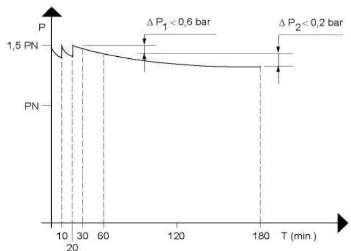
Figure 1 — Contrôle d'étanchéité
