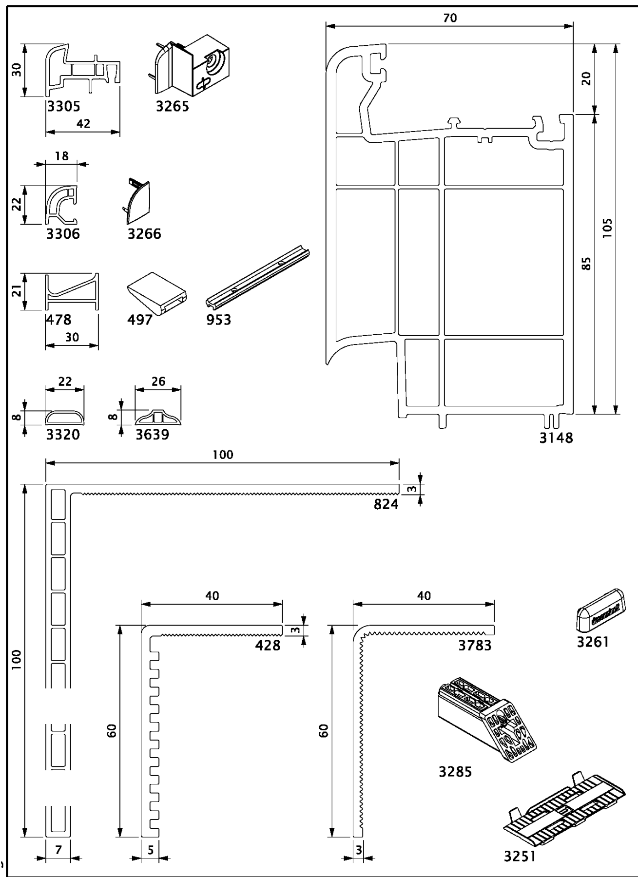
Figure 1i – Profils de finition
