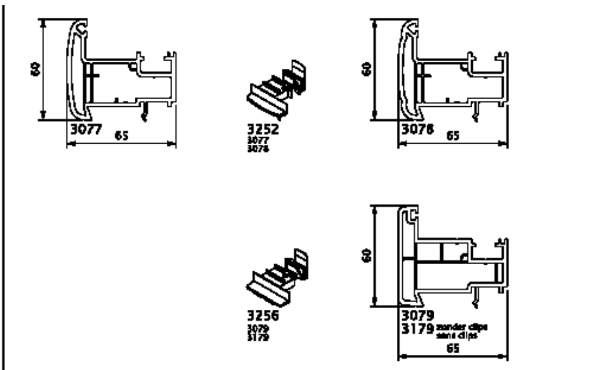
Figure 1e – Mauclairs et embouts pour mauclairs
