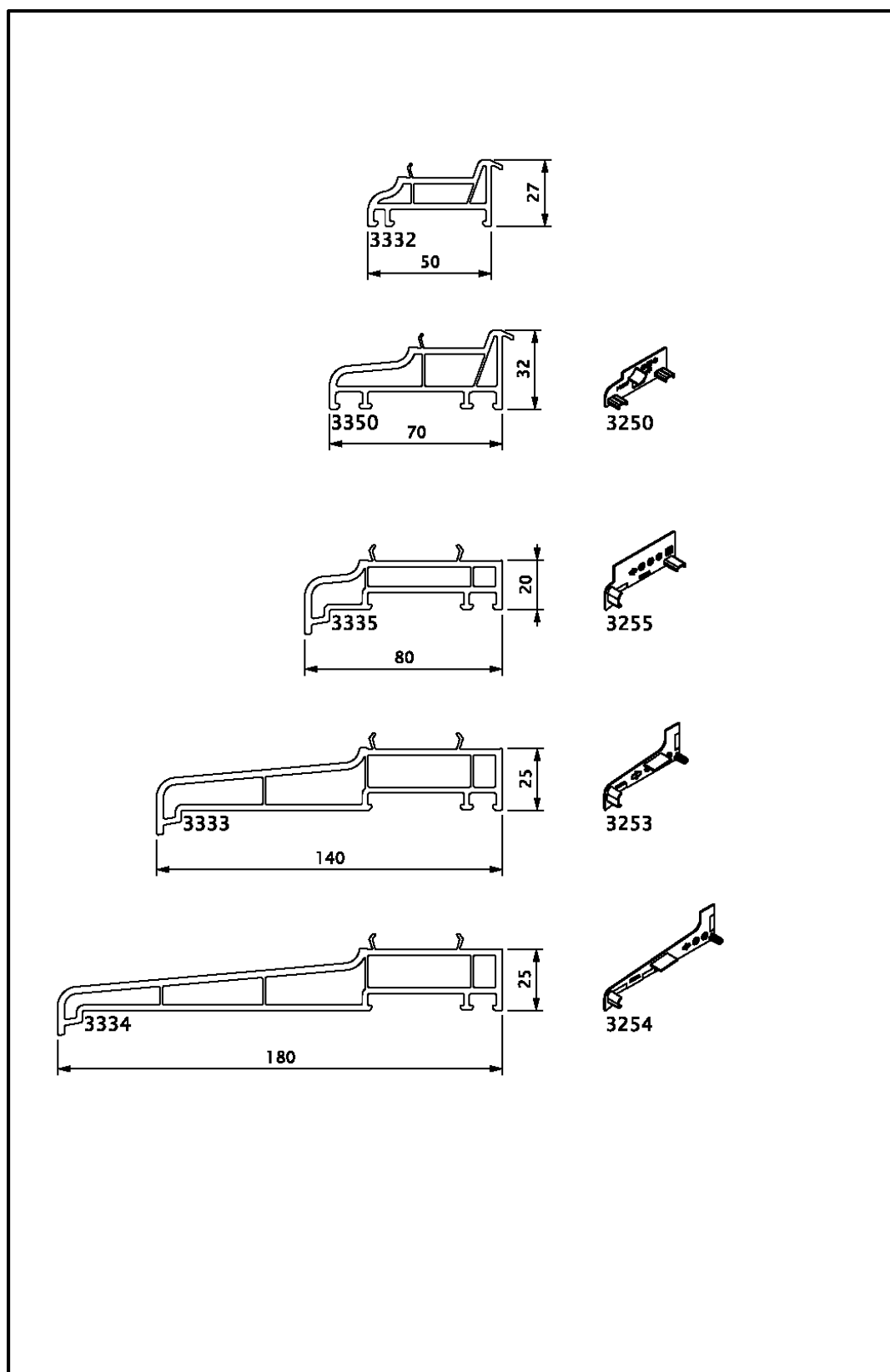
Figure 1h – Profils de seuil
