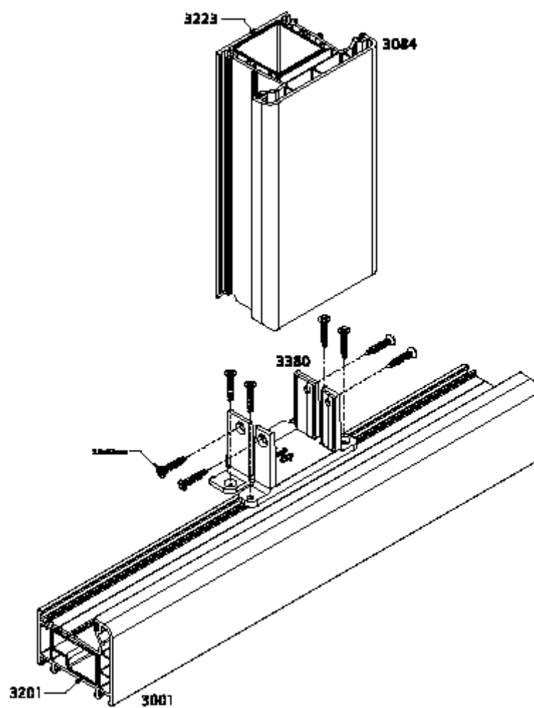
Figure 4b – Assemblage mécanique - type boulon ZAMAC
