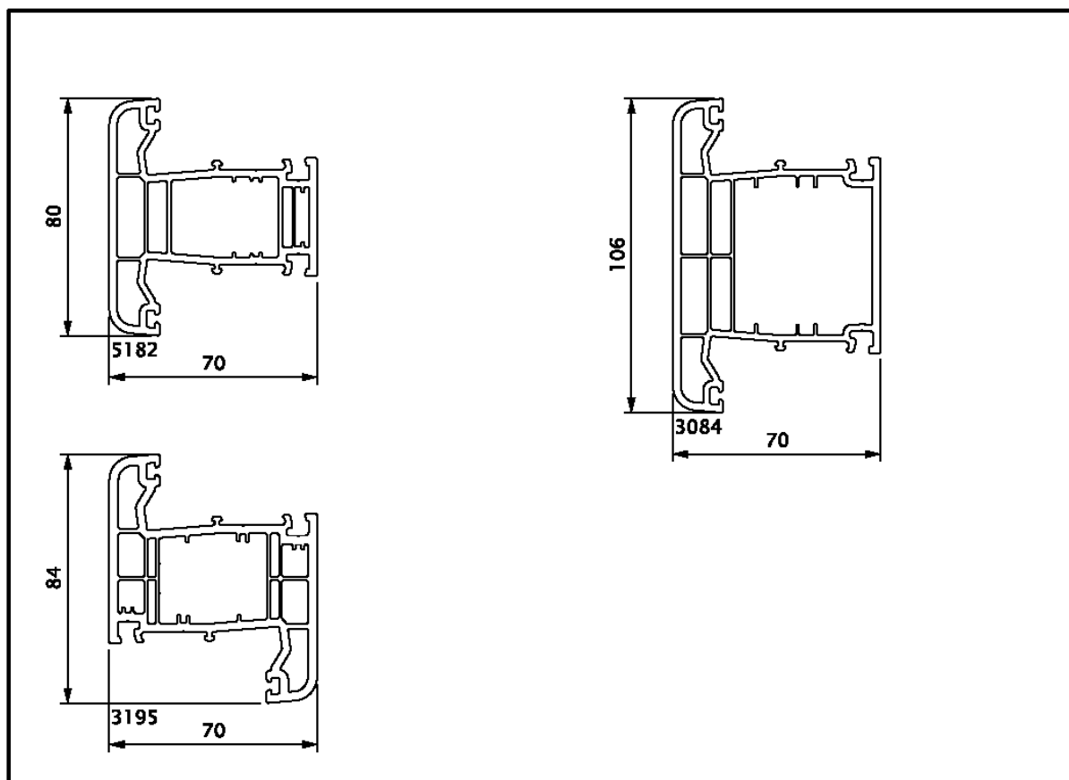
Figure 1e – Mauclairs et embouts pour mauclairs
