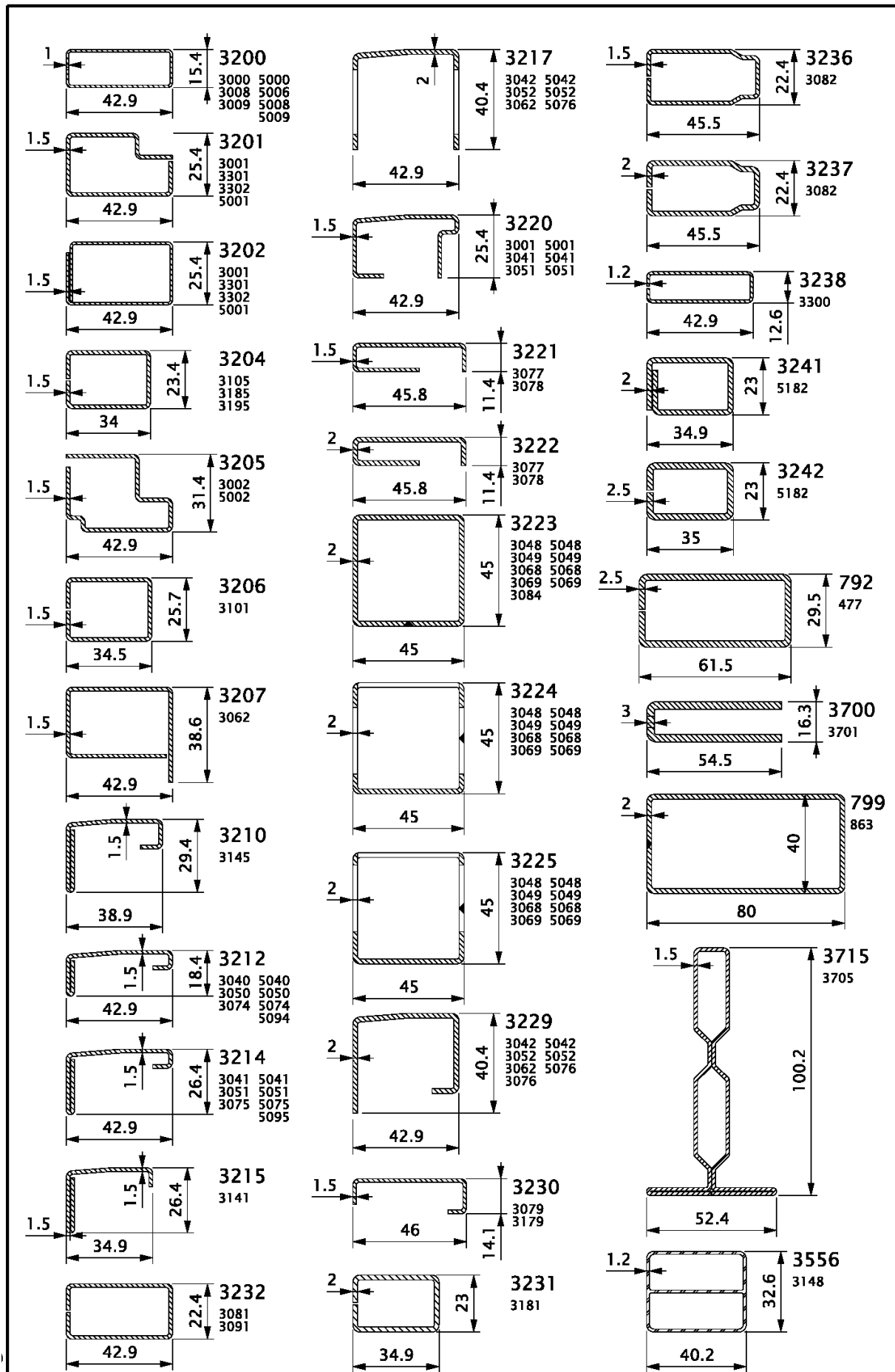
Figure 2 – Profils de renfort
