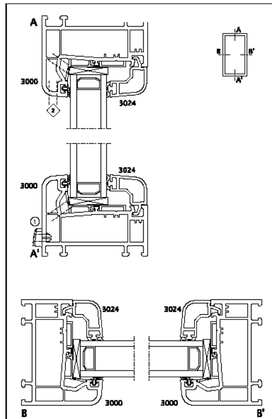
Figure 6 – Fenêtres à ouvrant et oscillo-battantes
