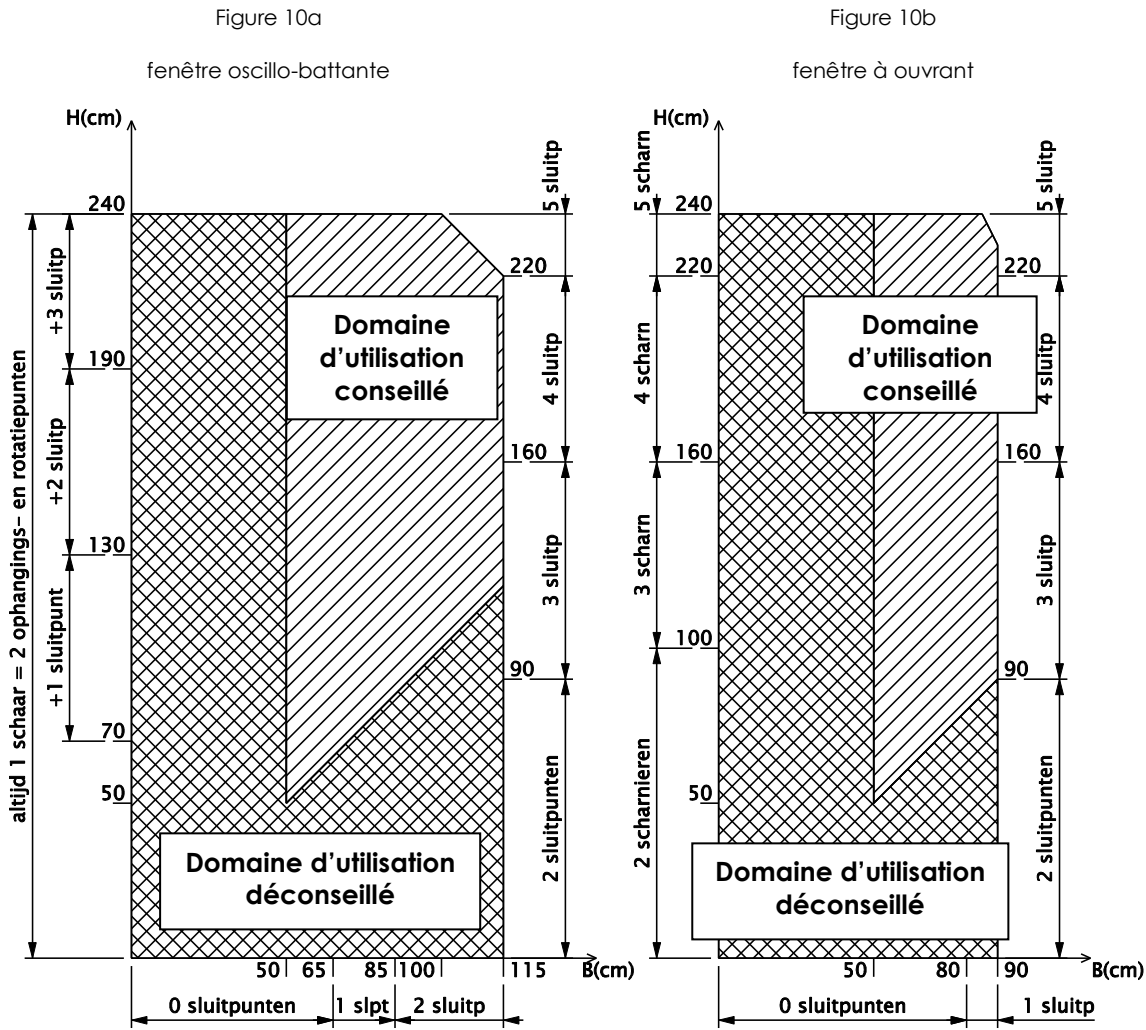
Figure 10 – Nombre de points de fermeture et de charnières en fonction des dimensions de l'ouvrant pour
