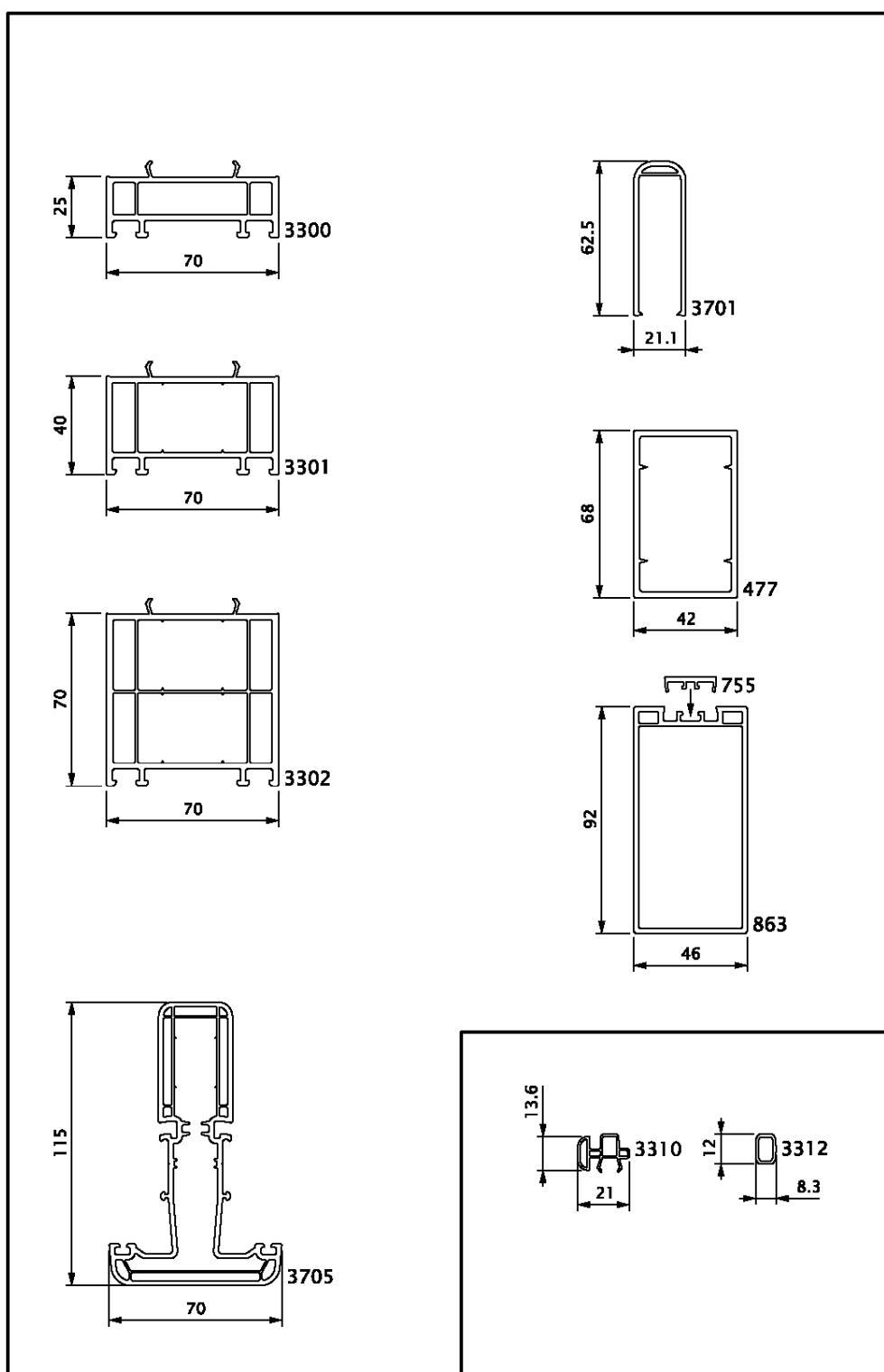
Figure 1b – Profilés d'assemblage
