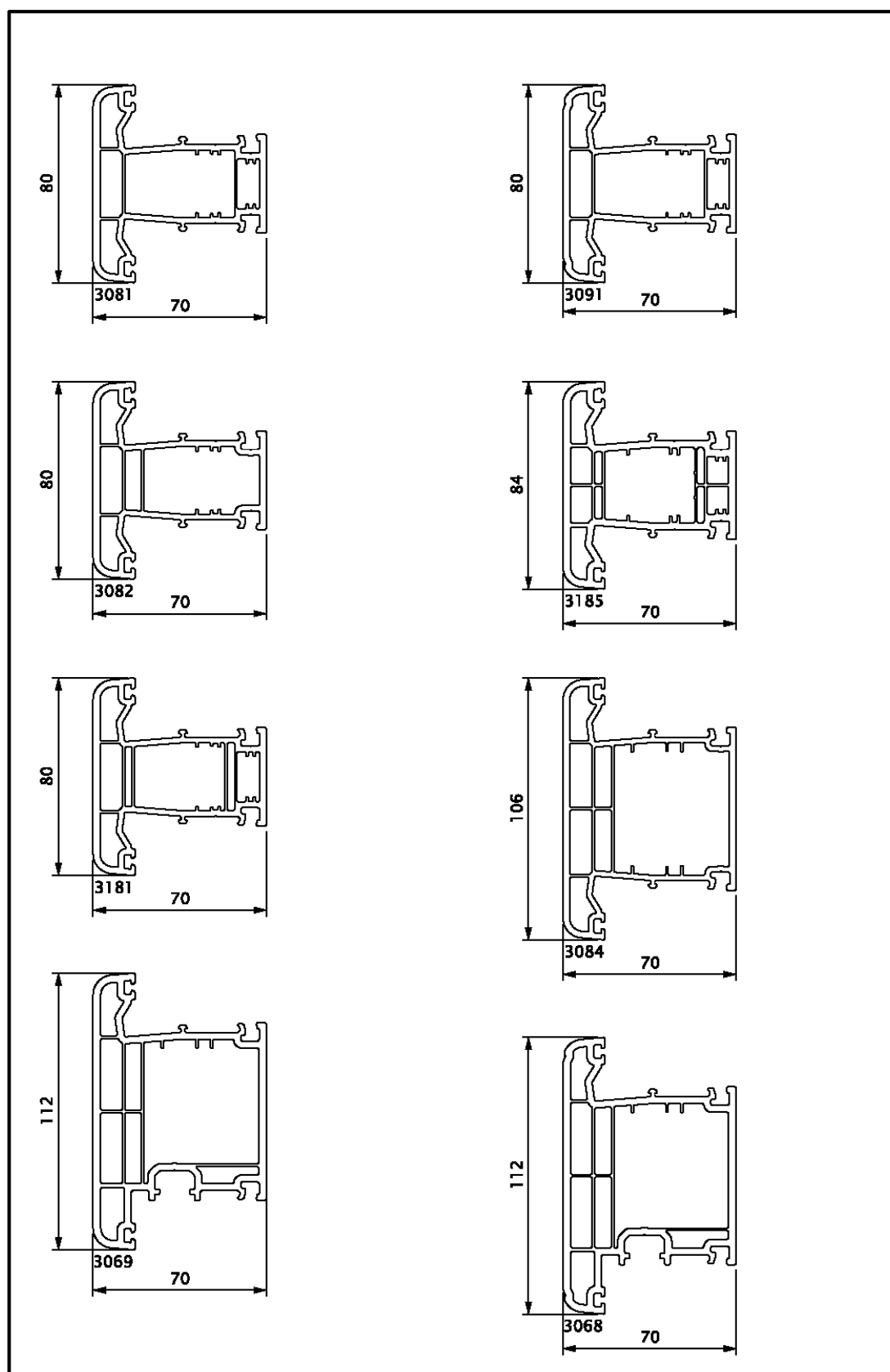
Figure 1d – Profilés de meneau ou de traverse
