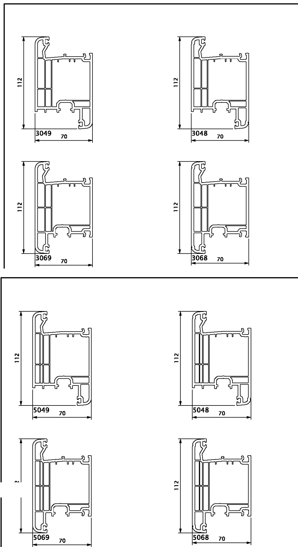
Figure 1c – Profilés d'ouvrant (suite)
