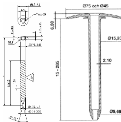
Fig. 2 – Schroef SFS ISOTAK® PS-48 + tule SFS ISOTAK® 45
