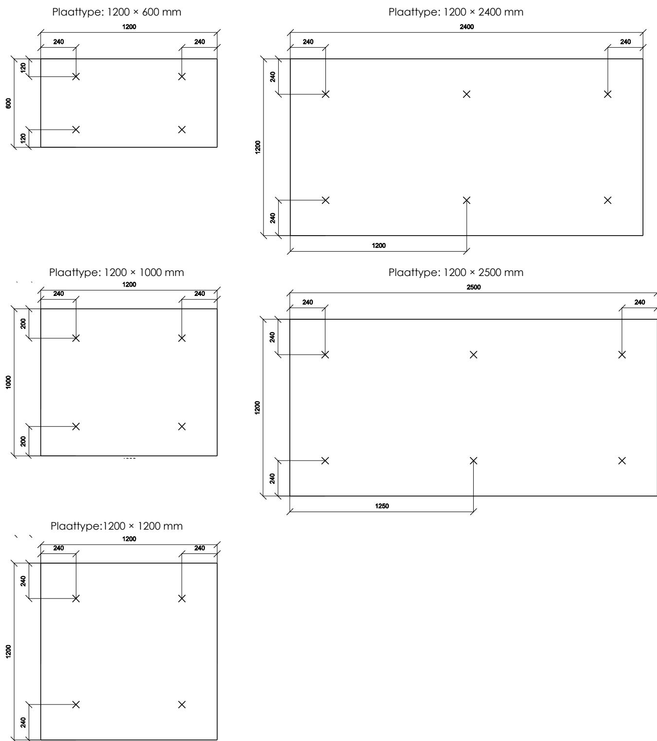
Fig. 1: plaatsingspatroon voor de mechanische bevestigingen
