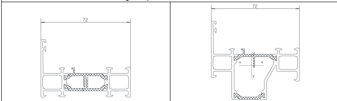
Figuur 4: Systeem RT 72 EN RT 72 REFLEX
