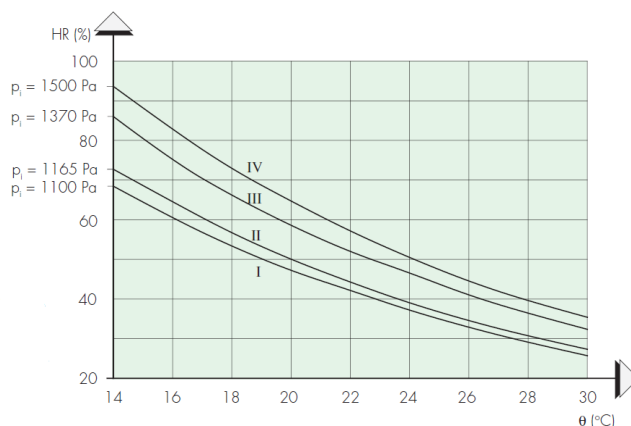
Fig. 1– Binnenklimaatklassen (jaargemiddelden)
