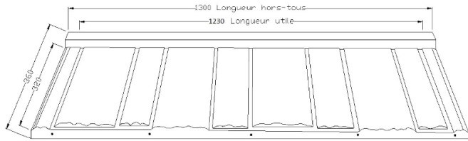
Fig. 3: tuile DECRA® STRATOS (ALZN)
