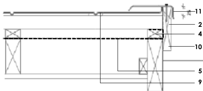
Fig. 15: Tuile QUADRO (ACOUSTIC) BY ICOPAL – réalisation du pied de versant avec profil de pied de versant
