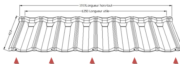
Fig. 7: tuile DECRA® OCTAVA (ALZN) – position des fixations
