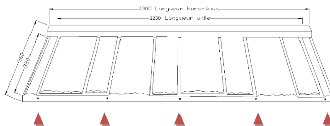
Fig. 8: tuile DECRA® STRATOS (ALZN) – position des fixations
