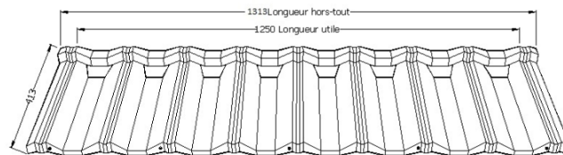
Fig. 2: tuile DECRA® OCTAVA (ALZN)
