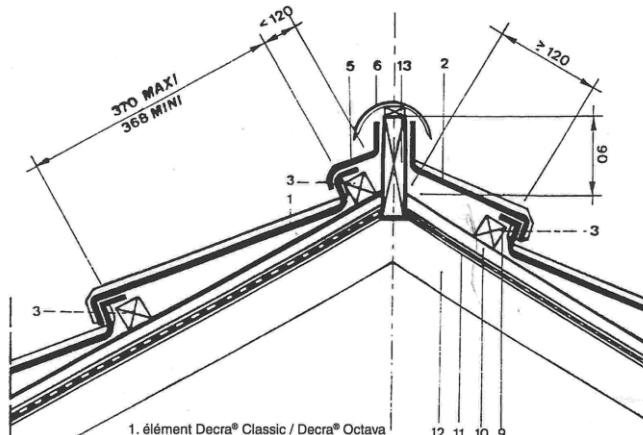
Fig. 10: tuile DECRA® CLASSIC (ALZN), DECRA® OCTAVA (ALZN), DECRA® STRATOS (ALZN) et DECRA® ELEGANCE – faîtière "V"
