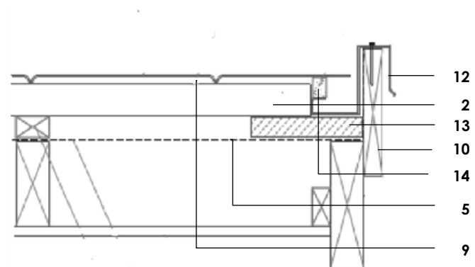
Fig. 17: Tuile QUADRO (ACOUSTIC) BY ICOPAL – rive latérale avec profil recouvrant la tuile
