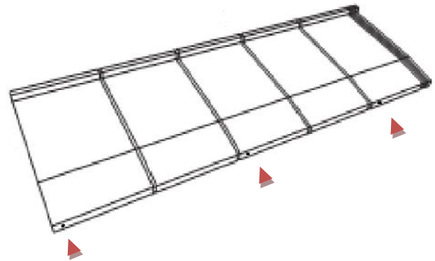
Fig. 13: tuile DECRA® QUADRO – position des fixations
