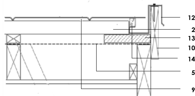
Fig. 17: Tuile QUADRO BY ICOPAL – rive latérale avec profil recouvrant la tuile
