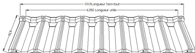
Fig. 2: tuile DECRA® OCTAVA
