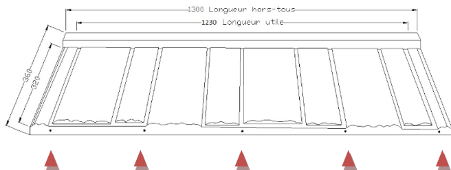
Fig. 8: tuile DECRA® STRATOS – position des fixations
