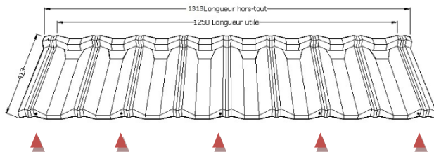
Fig. 7: tuile DECRA® OCTAVA – position des fixations
