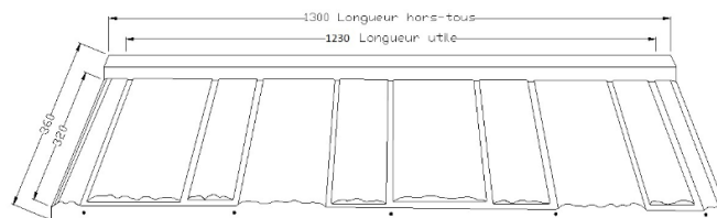
Fig. 3: tuile DECRA® STRATOS
