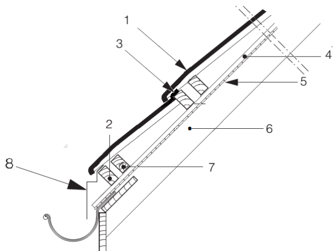
Fig. 14: Tuile QUADRO BY ICOPAL – réalisation du pied de versant avec élément entier finissant dans la gouttière
