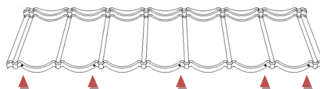
Fig. 5 – BMI AERODEK® TRADITION (PLUS), BMI AERODEK® UNIQUE PLUS P dakpannen – positie van de bevestigingen
