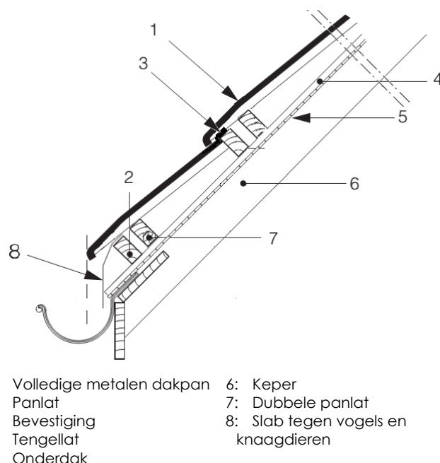
Fig. 12 – BMI AERODEK® QUADRO PLUS P dakpannen – uitvoering van de dakvoet met volledig element eindigend in de dakgoot
