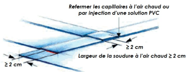
Fig. 5 – Mise en œuvre des joints en T (soudage à l'air chaud)
