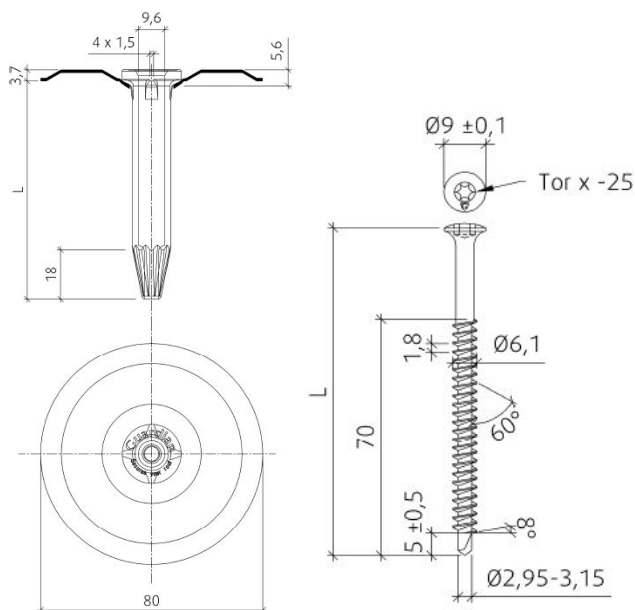
Fig. 4 – vis GUARDIAN® BS 6,1 + plaquette GUARDIAN® GWSP-80-F2E + tule GUARDIAN® GWT
