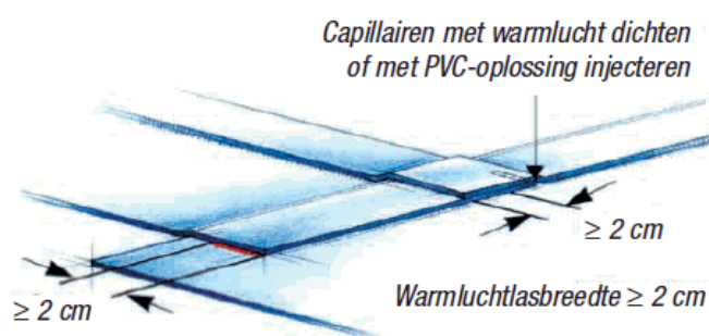
Fig. 5 – Verwerking T-naden
