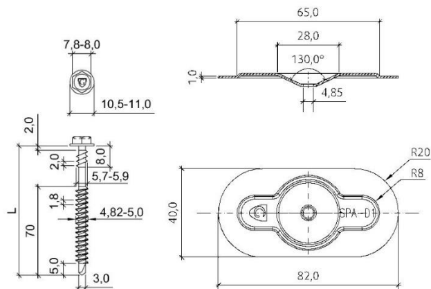
Fig. 2 – Guardian systeem – schroef & plaatje
