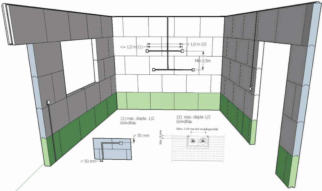
Figuur 5: in acht te nemen afstanden bij het inwerken van leidingen
