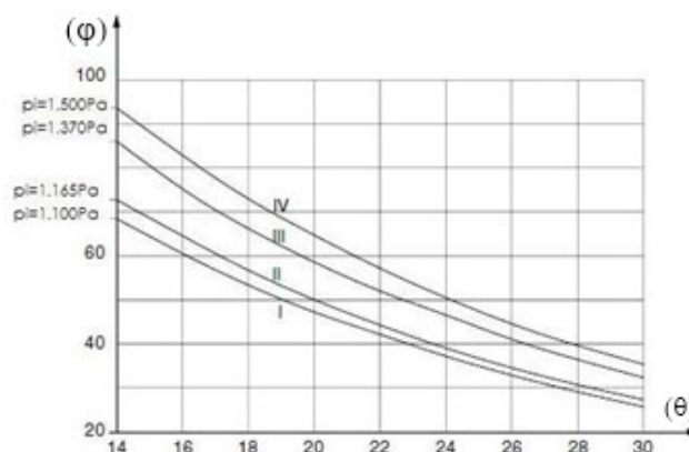
Grafiek – Binnenklimaatklassen (jaargemiddelden)
