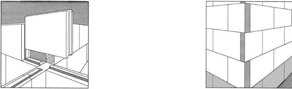
Figuur 4a: een koker gebouwd met gipsblokken
