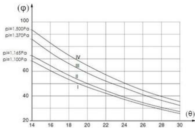
Grafiek – Binnenklimaatklassen (jaargemiddelden)
