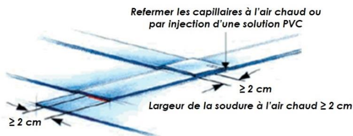
Fig. 1: Mise en œuvre des joints en T
