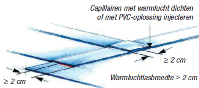
Fig. 1 – Verwerking T-naden bij lassen met hete lucht
