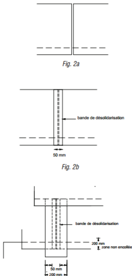
Fig. 2 – Recouvrement des lés (transversal)
