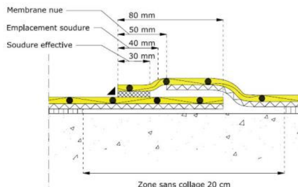
Fig. 1 – Recouvrement des lés (longitudinal)
