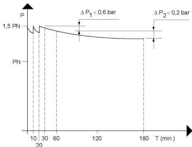
Fig. 2: Contrôle d'étanchéité
