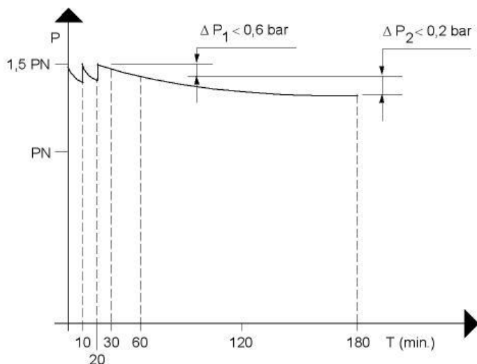
Fig. 2: Dichtheidscontrole
