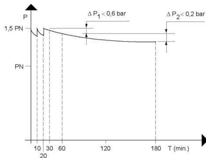
Fig. 4: Contrôle d'étanchéité
