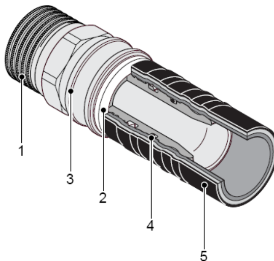
Fig. 1: Doorsnede Geberit MEPLA perskoppelstuk
