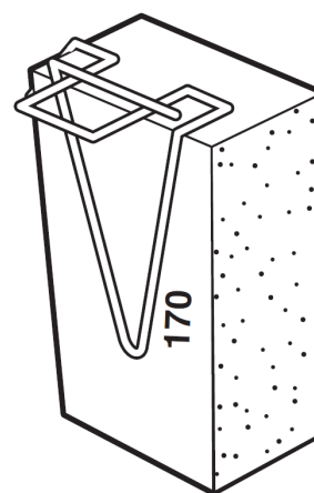
Fig. 4 – Murfor® Lateihaak (LKH/S-170)
