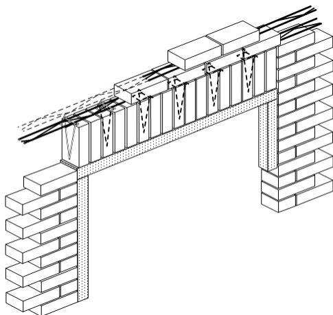
Fig. 9 – Positionering van de lateihaken
