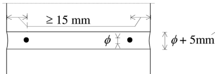
Fig. 5 – Positionering van de lintvoegwapening in de voeg
