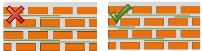
Fig. 8 – Verspringen van Murfor® elementen
