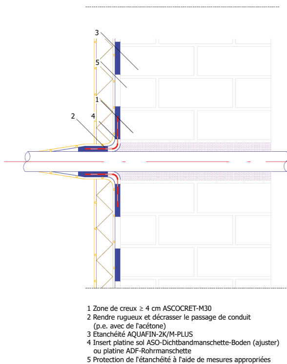
Fig. 6 – Scellement d'un passage de conduit à l'aide d'AQUAFIN-2K/M-PLUS
