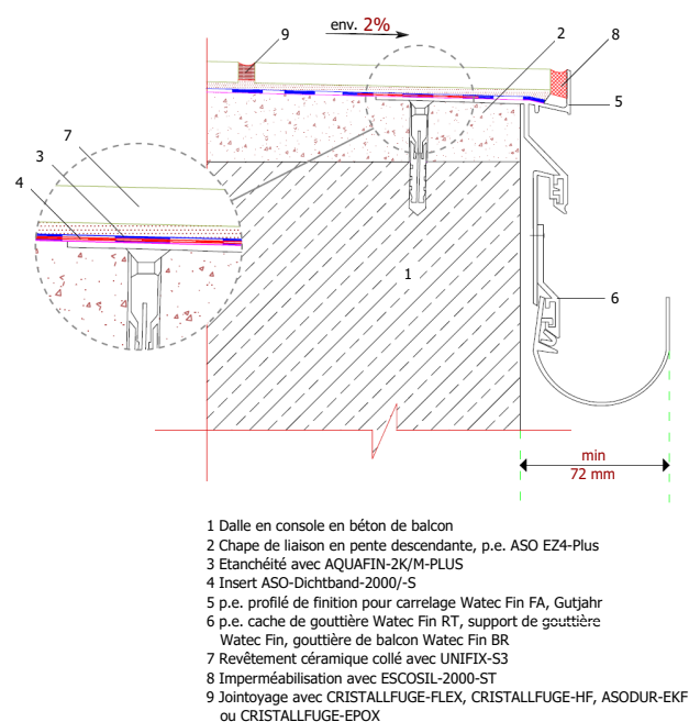
Fig. 4 – Scellement de balcon à l'aide d'AQUAFIN-2K/M-PLUS, bord de balcon avec rigole
