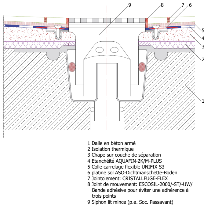
Fig. 9 – Scellement d'un siphon de sol en pièce humide à l'aide d'AQUAFIN-2K/M-PLUS
