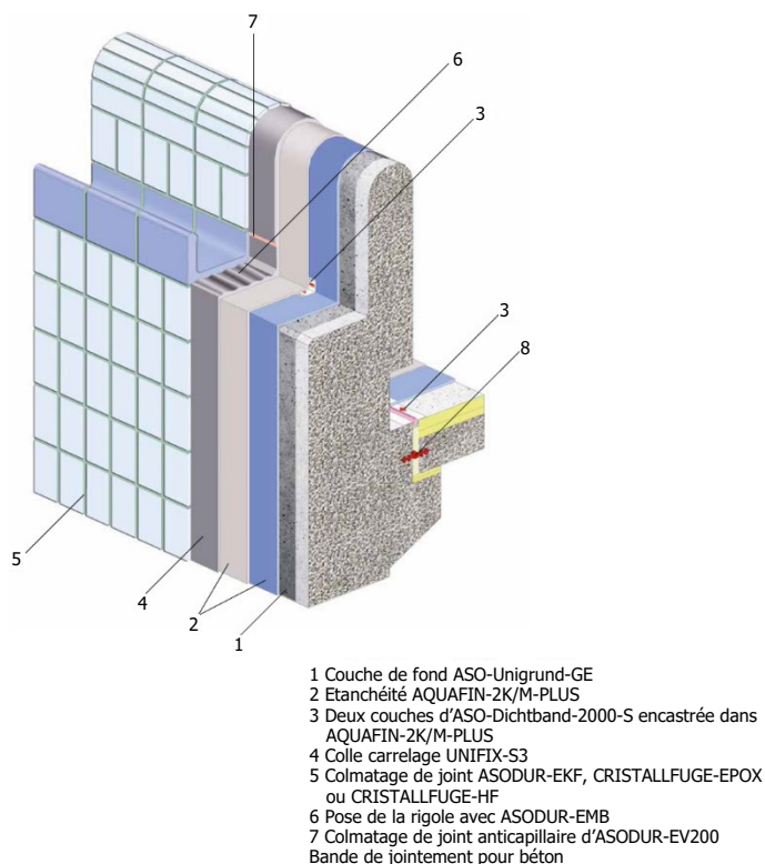
Fig. 12 – Rigole type Wiesbaden, sollicitation par de l'eau sous pression à l'intérieur ou à l'extérieur
