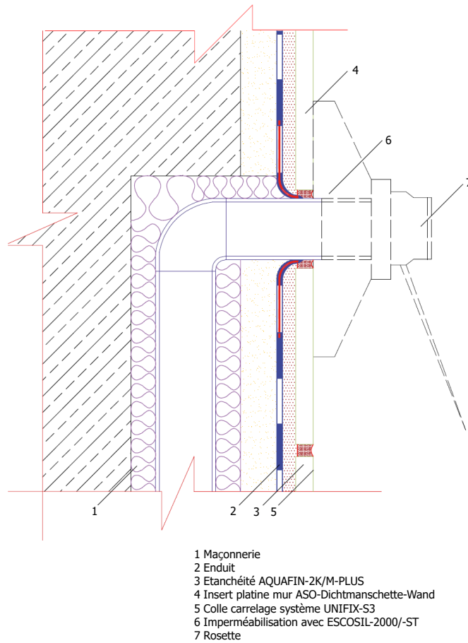
Fig. 8 – Scellement d'un passage de conduit en pièces humides, sollicitation par de l'eau sans pression à l'intérieur
