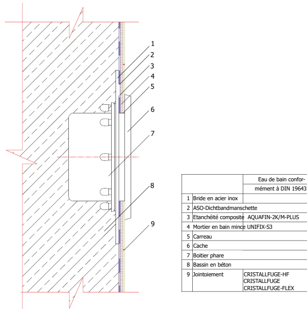
Fig. 10 – Étanchéité de de phares sous-marins avec brides
