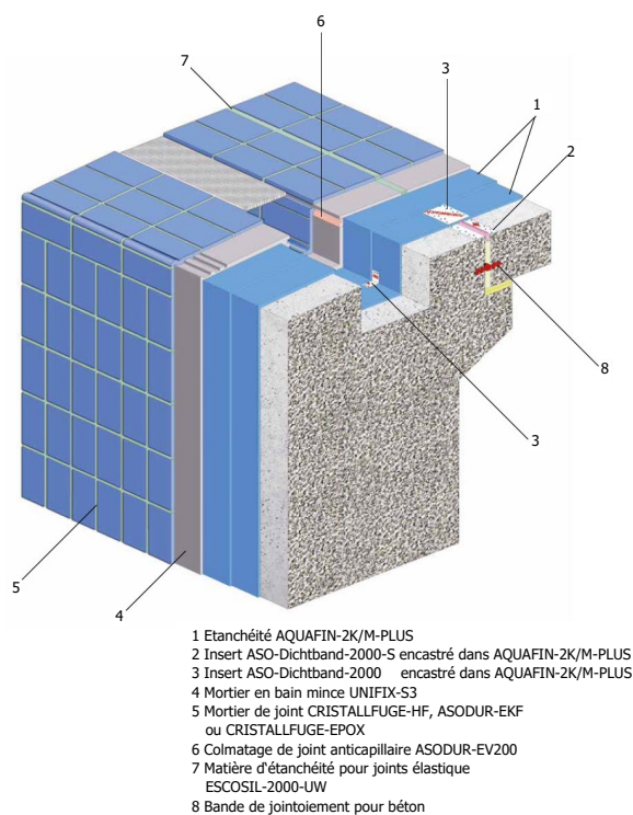
Fig. 13 – Carreau anti-dérapant, sollicitation par de l'eau sous pression à l'intérieur ou à l'extérieur
