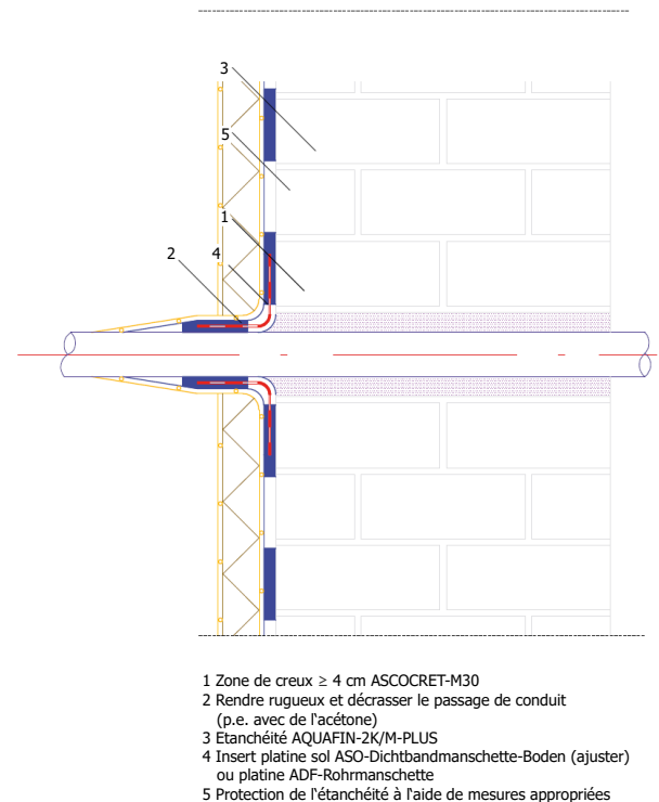
Fig. 6 – Scellement d'un passage de conduit à l'aide d'AQUAFIN-2K/M-PLUS
