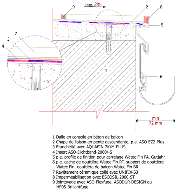
Fig. 4 – Scellement de balcon à l'aide d'AQUAFIN-2K/M-PLUS, bord de balcon avec rigole
