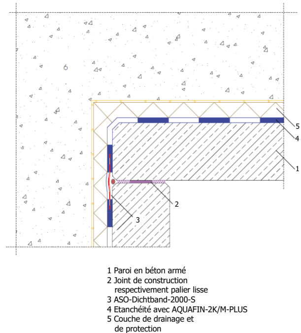
Fig. 2 – Etanchéité d'un joint de construction respectivement d'un palier lisse à l'aide d'AQUAFIN-2K/M-PLUS
