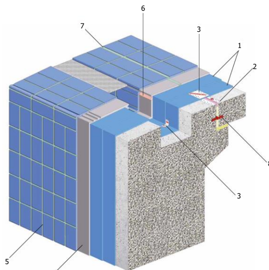
Fig. 12 – Rigole type Wiesbaden, sollicitation par de l'eau sous pression à l'intérieur ou à l'extérieur
