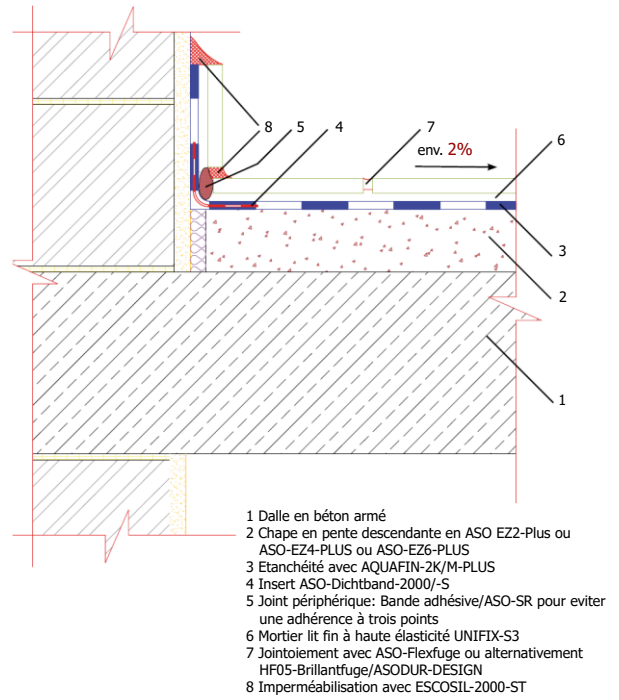
Fig. 5: Etanchéité de balcon avec AQUAFIN-2K/M-PLUS, raccord paroi/sol, sollicitation par de l'eau sans pression à l'extérieur
