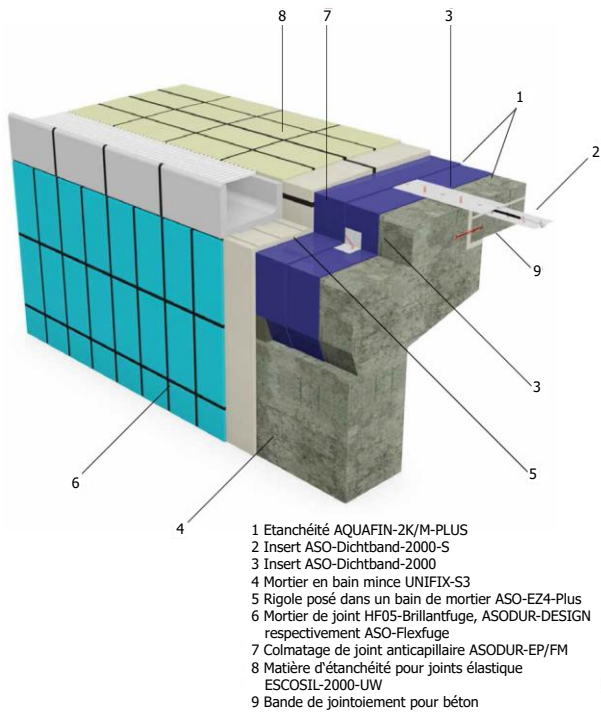
Fig. 14: Etanchéité pour bassins thérapeutiques, propriétés d'eau potable, sollicitation par de l'eau sous pression à l'intérieur ou à l'extérieur
