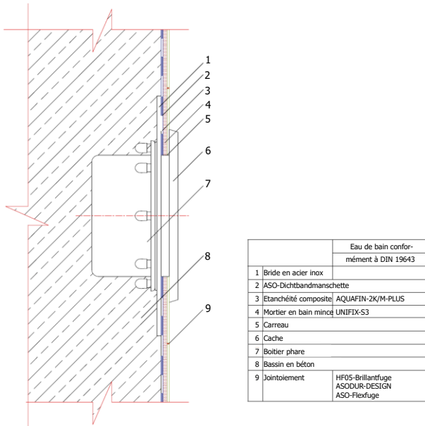
Fig. 10: Etanchéité de de phares sous-marins avec brides
