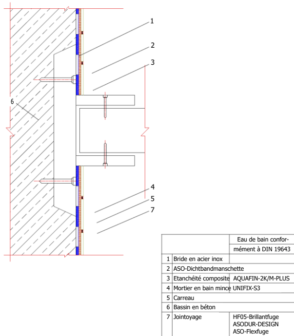
Fig. 11: Bride de scellement pour pièce à insérer
