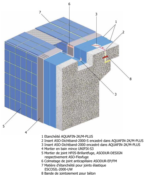
Fig. 13: Carreau anti-dérapant, sollicitation par de l'eau sous pression à l'intérieur ou à l'extérieur
