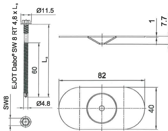
Fig. 3 – Vis EJOT SW8-RT-4,8 + plaque de fixation EJOT HTV 82/40 F
