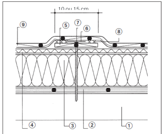
Fig. 7 – Fixation au moyen de bandes distinctes
