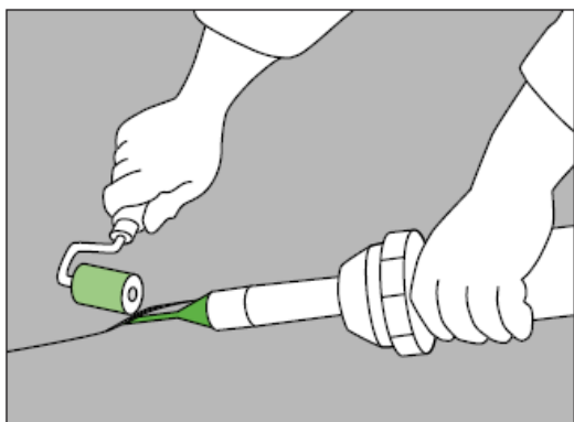
Fig. 8 – Recouvrement des lés (à l'air chaud)
