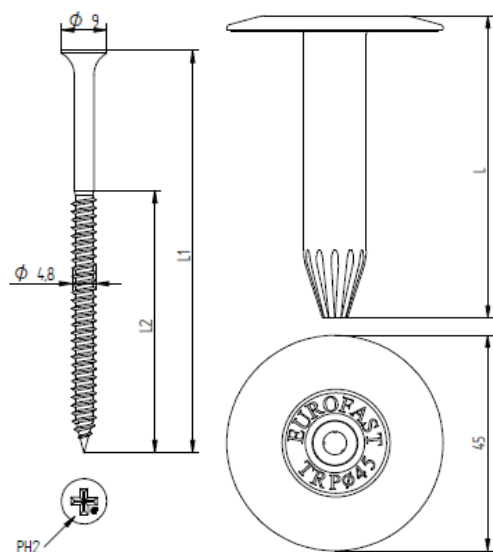
Fig. 1 – Vis EUROFAST EDS-S-48 + tube télescopique EUROFAST TRP-45
