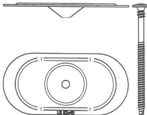
Fig. 1 – ETANCO EVB DF 2C et plaquelette 82x40 R
