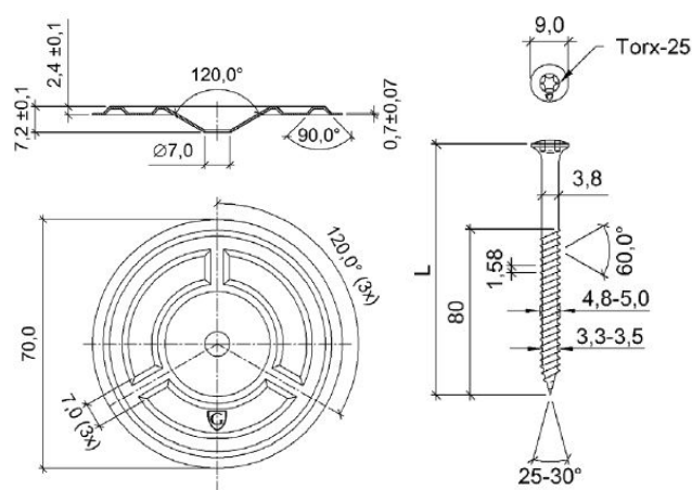
Fig. 2 – GUARDIAN PS 4,8 et plaquelette GUARDIAN SP-70-S
