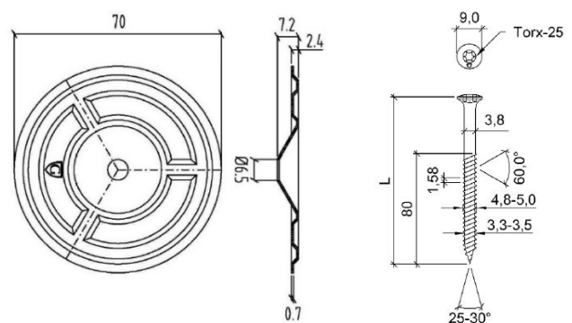
Fig. 1 – Vis GUARDIAN PS 4,8 et plaquelette GUARDIAN SP-70-S
