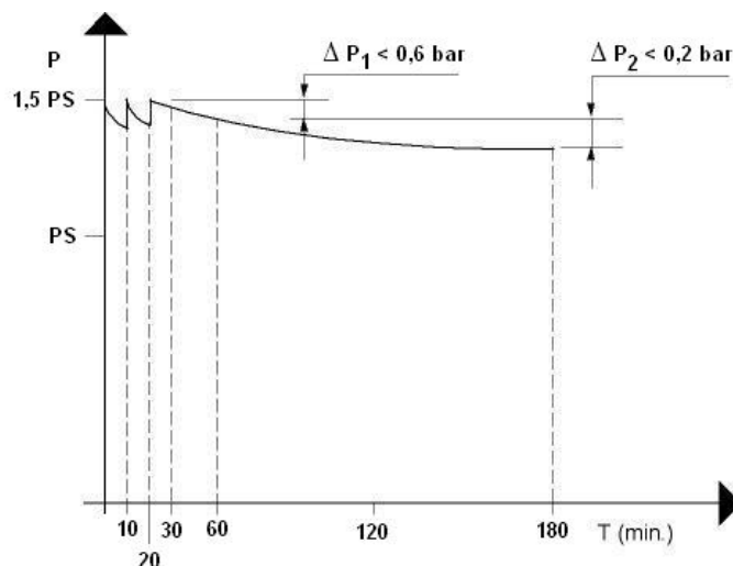
Fig. 1 Procedure dichtheidscontrole
